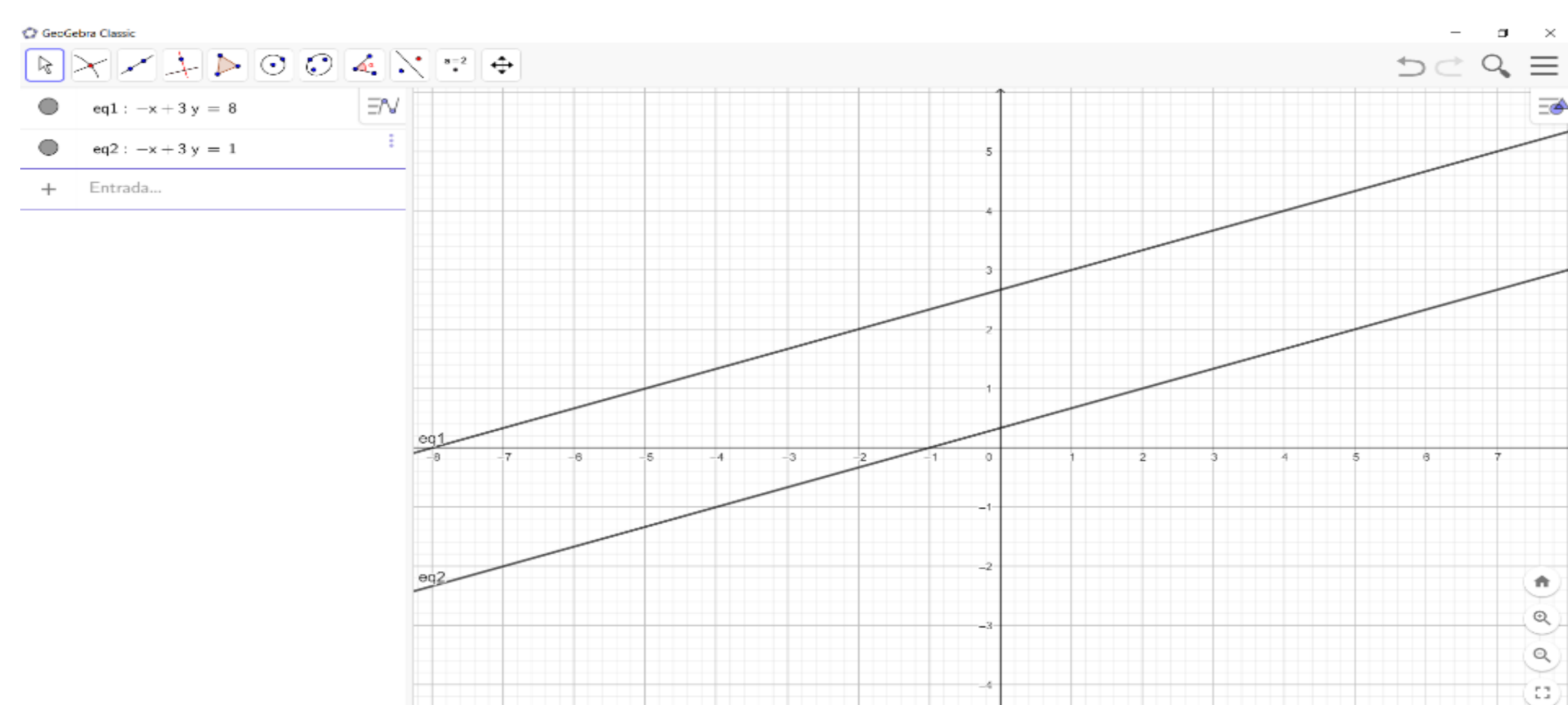
Figura 2: Retas Paralelas
