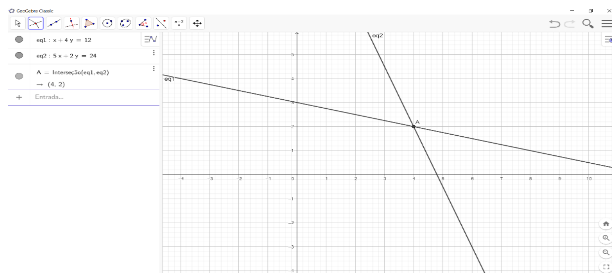
Figura 1: Retas Concorrentes
