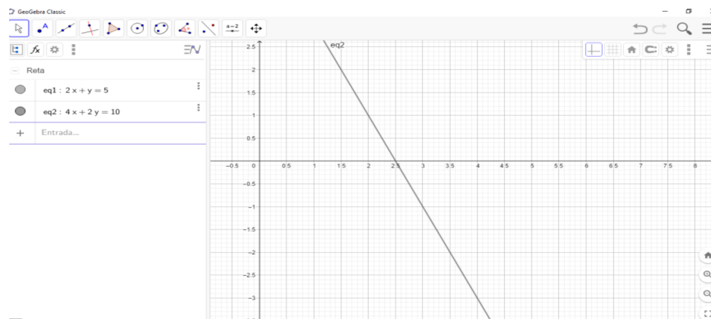
Figura 3: Retas Coincidentes
